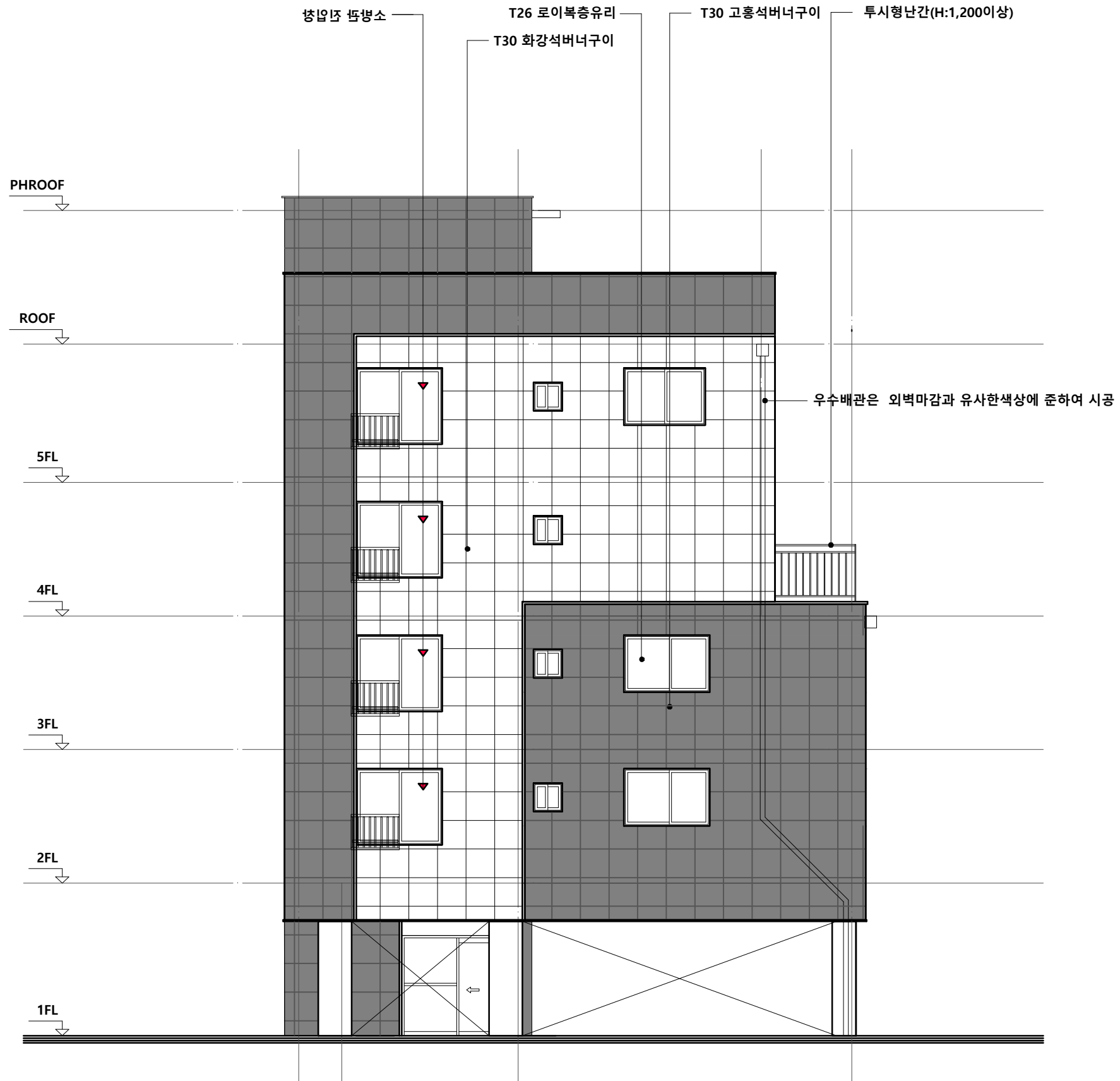
정 면 도 1 SCALE : 1/100
